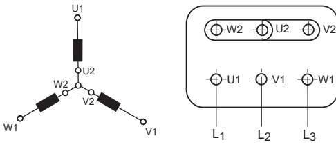
Рис. 11 Соединение звездой
