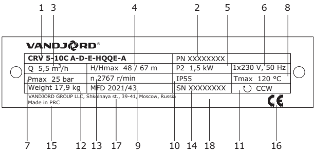
Рис. 2 Фирменная табличка
