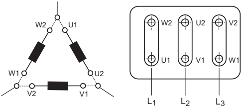
Рис. 10 Соединение треугольником
