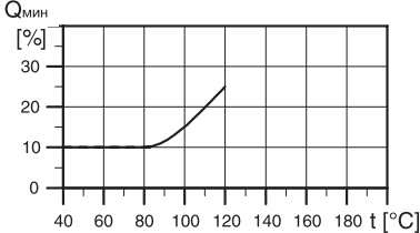
Рис. 20 Минимальная подача
