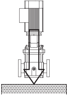
Рис. 4 Правильный монтаж
