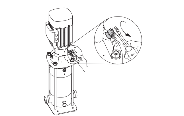
Рис. 16 Воздуховыпускной клапан
